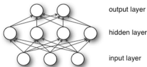
图 1. 多层感知机模型
